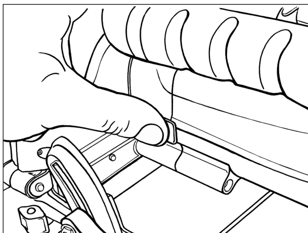
Рис.9 Блокировка шпинделя
