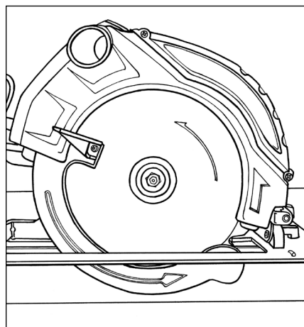
Рис.6 Установка глубины
