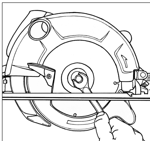
Рис.10 Откручивание болта
