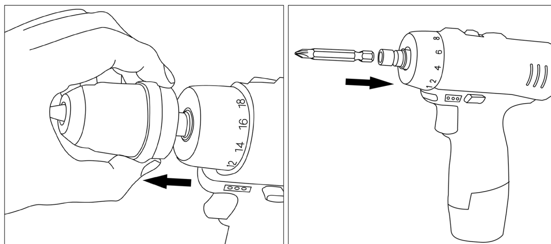
Рис. 9 Быстросъемный патрон.
