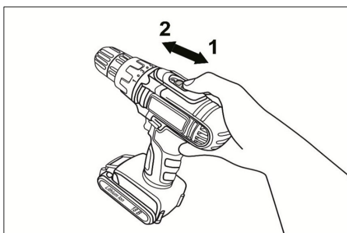
Рис. 13 Переключение скоростей
