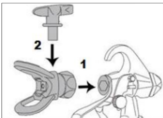
Рис. 8. Установка соплодержателя и сопла
