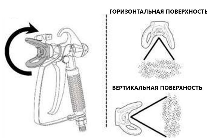
Рис. 21. Поворот соплодержателя
