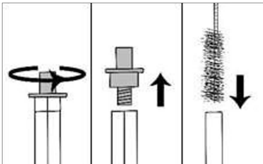
Рис. 26. Очистка сетчатого фильтра
