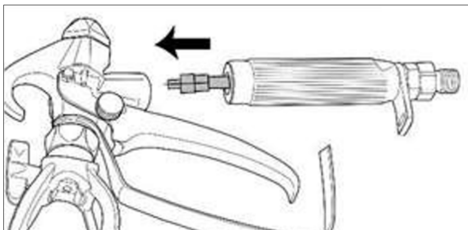
Рис. 24. Снятие фильтра
