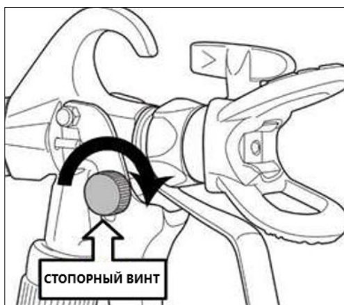
Рис. 11. Блокировка пистолета распылителя
