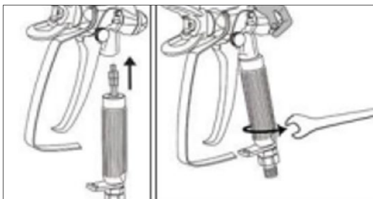
Рис. 5. Установка фильтра в пистолет-распылитель
