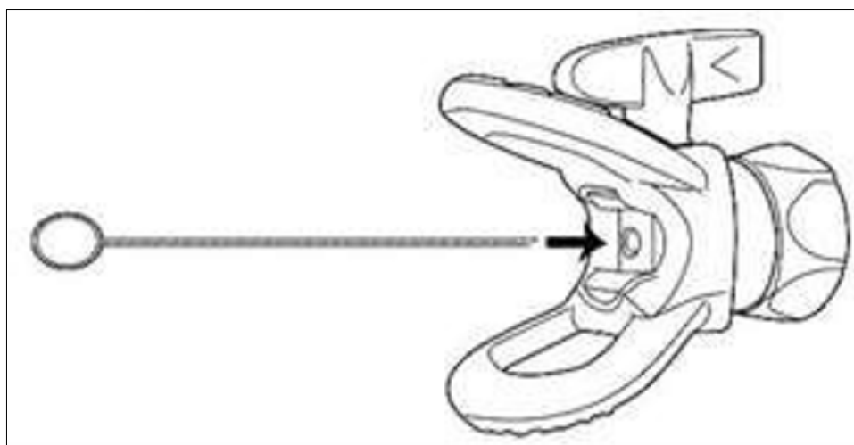
Рис. 25. Очистка сопла
